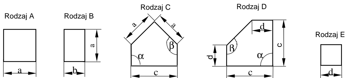
Rysunek 1. Rodzaje płyt chodnikowych betonowych
